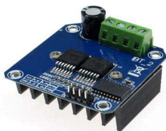
图3 电机驱动模块 BTS7960
